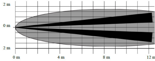
Vista dall'alto installazione a corridoio
